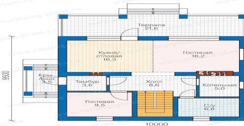
План первого этажа
