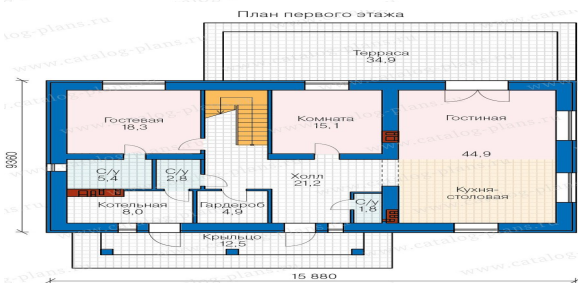
План первого этажа
