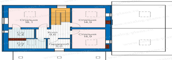
План мансардного этажа
