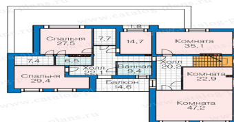
План второго этажа
