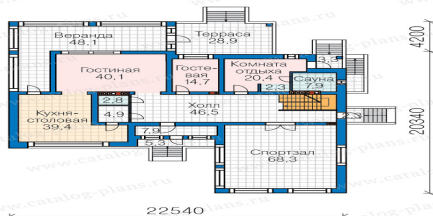
План первого этажа
