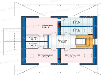
План второго этажа
