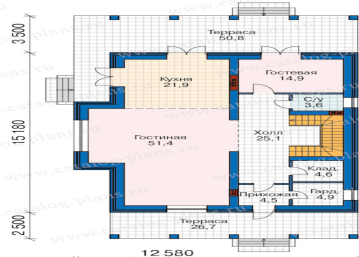
План первого этажа
