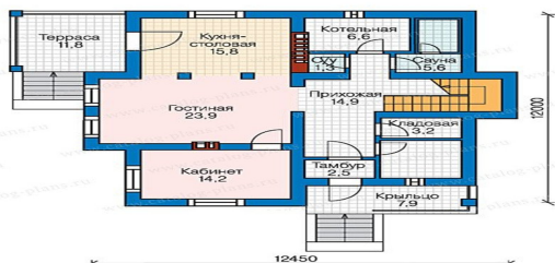
План первого этажа
