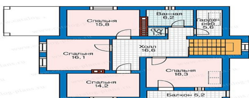
План второго этажа
