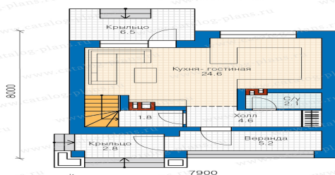
План первого этажа
