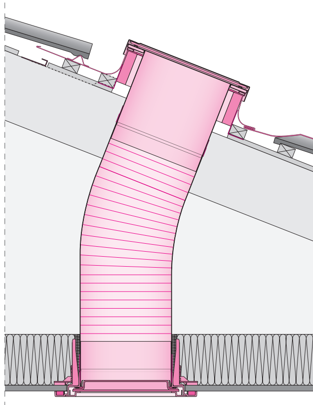
Сечение Туннеля дневного света SF_
