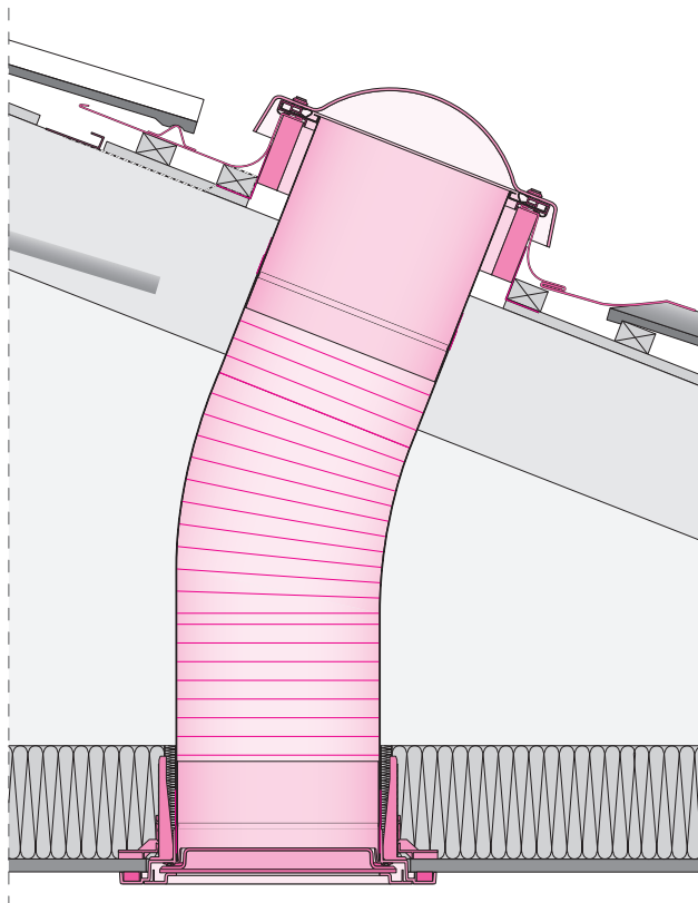
Сечение Туннеля дневного света SFD
